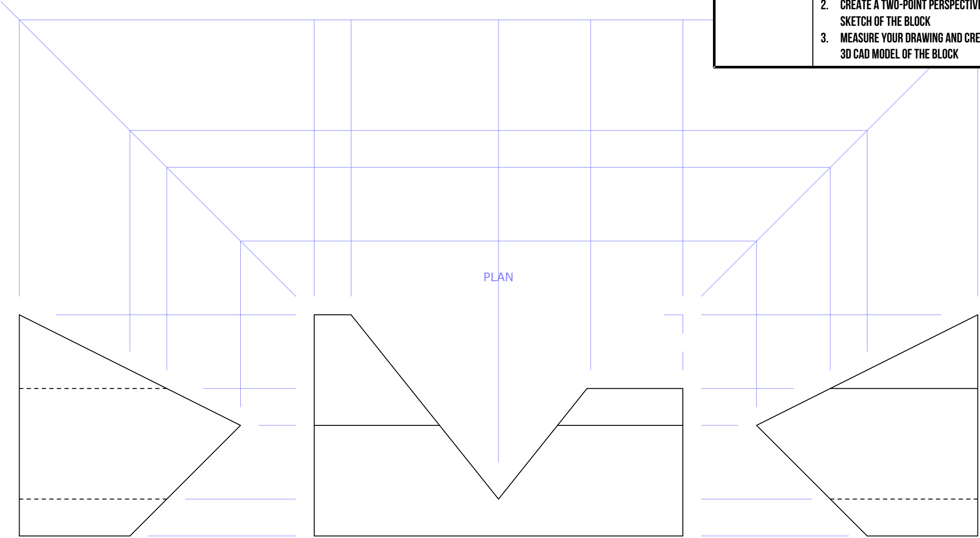
END ELEVATION
