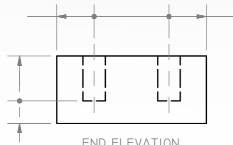
END ELEVATION
